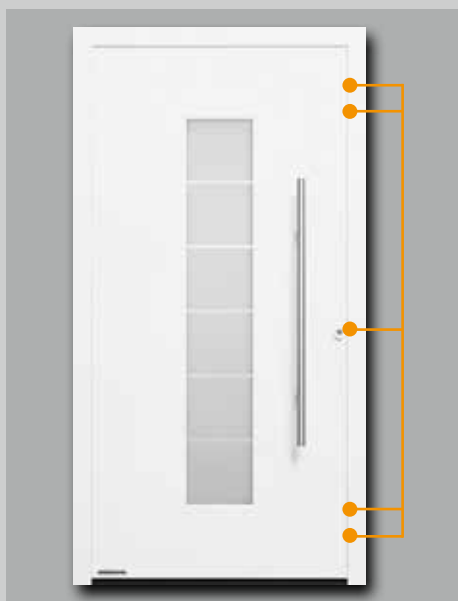
Serrure de sécurité 5 points H5 avec têtère en acier inoxydable
